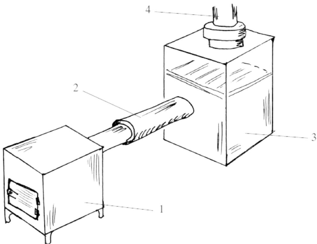
Рис. 10. Коптильня из старого холодильника:
