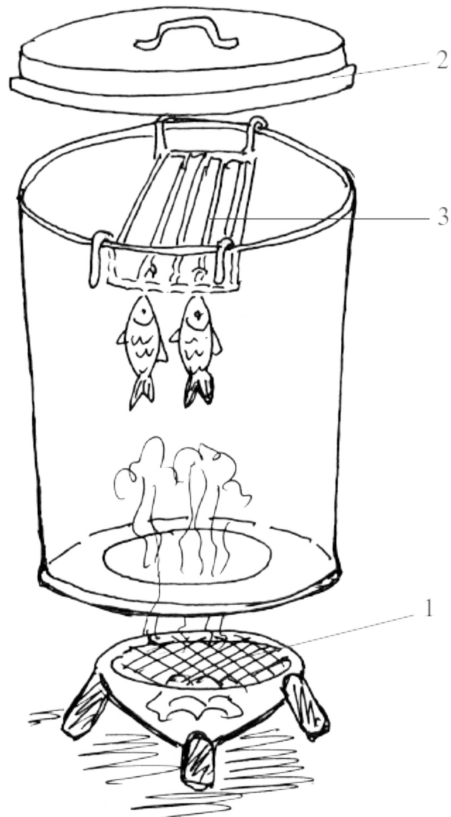
Рис. 4. Коптильня из бака:
