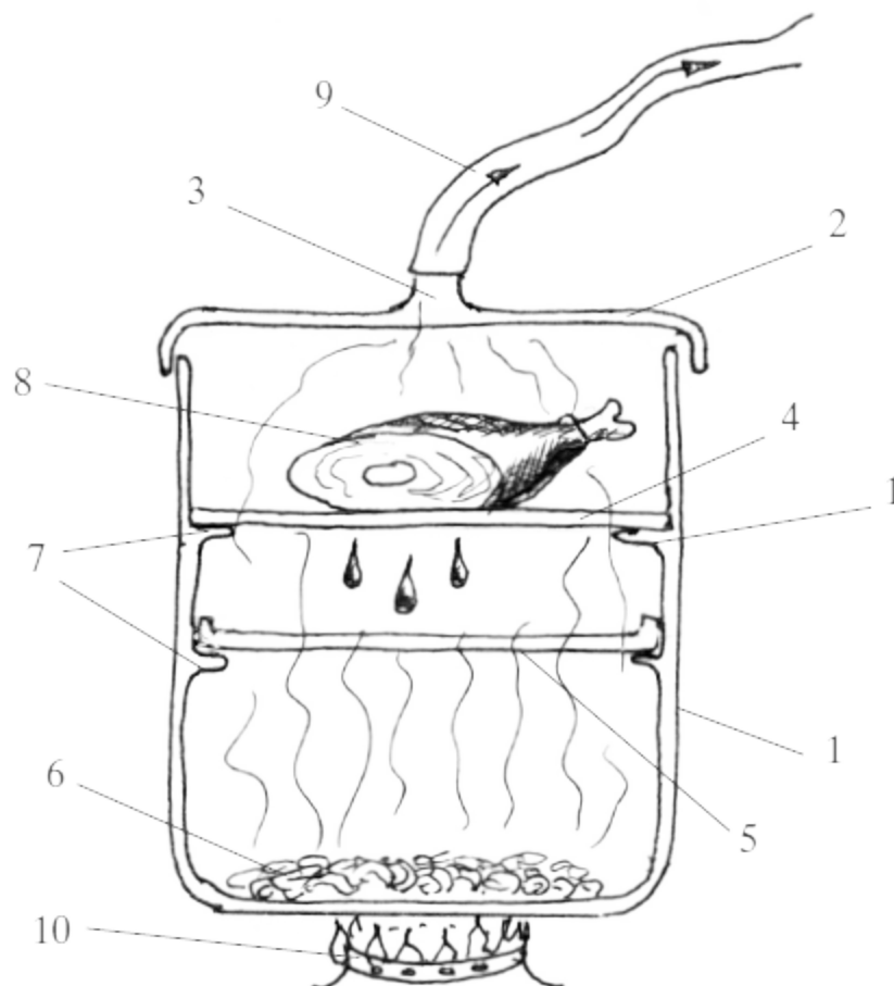
Рис. 11. Копчение на плите в квартире:
