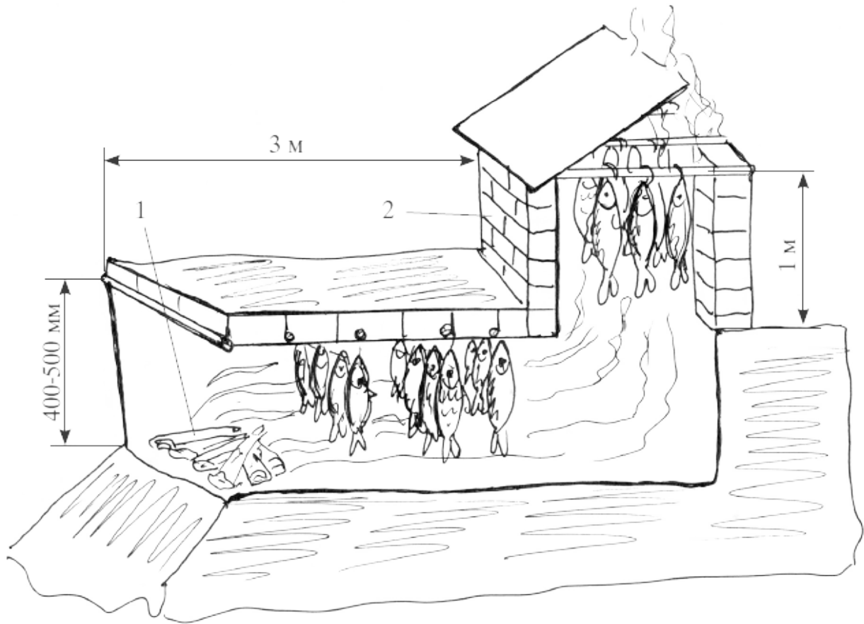
Рис. 8. Стационарная коптильня в земле: 1 – костер; 2 – коптильная камера
