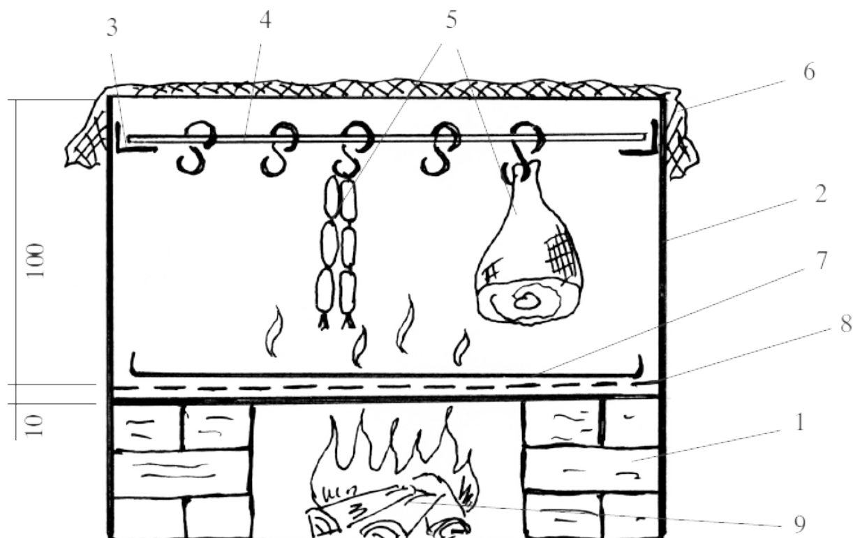
Рис. 1. Простейшая коптильня из железного ящика:
