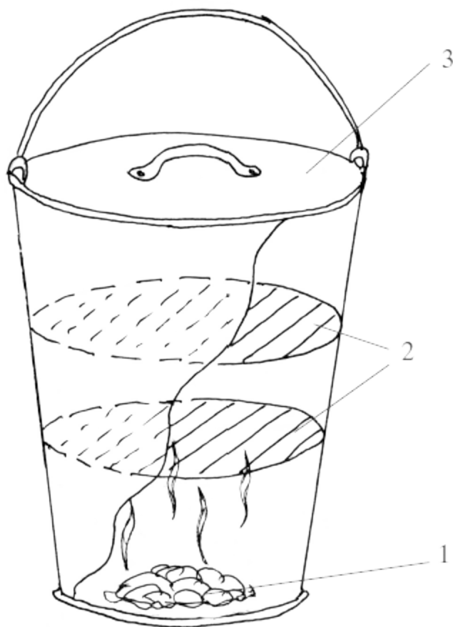
Рис. 6. Коптильня из ведра:
